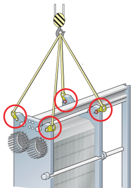
Slika 7: Dvižna naprava za AQ18 in AQ14L. Pritrdilna oprema ni potrebna.
