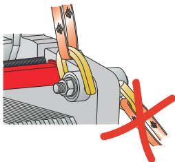
Slika 9: Dvižna naprava za AQ20S. Pri dvigovanju ploščnega izmenjevalnika toplote uporabite štiri notranje oči. NE uporabljajte točk za zavarovanje med transportom! Pritrdilna oprema je potrebna.
