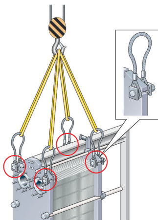
Slika 6: Dvižna naprava za AQ14 in AQ14S. Pritrdilna oprema je potrebna.
