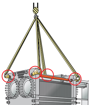
Slika 8: Dvižna naprava za AQ20. Pritrdilna oprema je potrebna.
